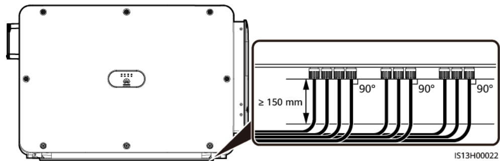
Abbildung 5-18 Anschlussanforderungen für DC-Eingangstromkabel
