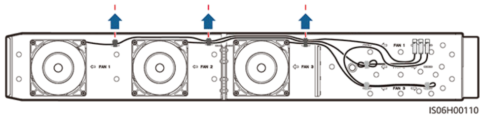
Abbildung 8-6 Entfernen der Kabelbinder für LÜFTER 1
