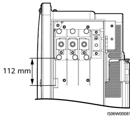
Abbildung 5-10 Spezifikationen der Gummischutzplatte
