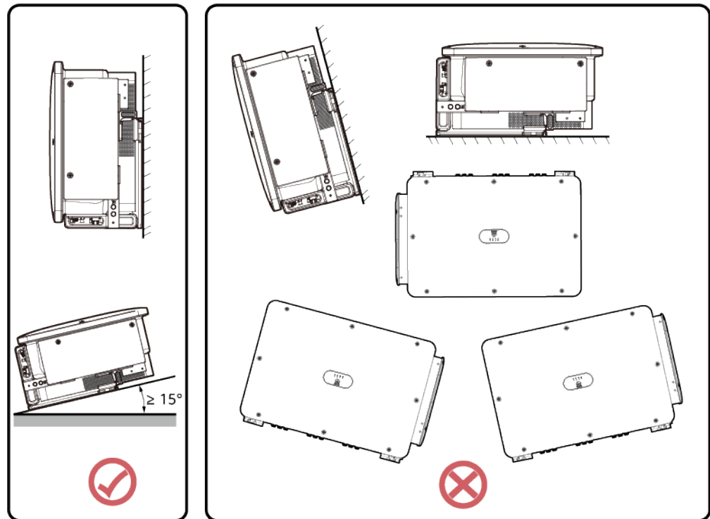
Abbildung 4-3 Montagewinkel
