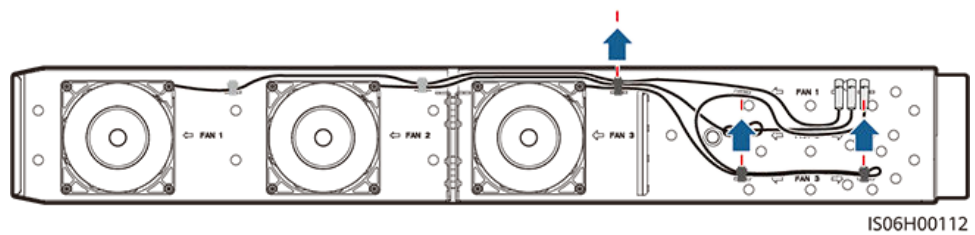
Abbildung 8-8 Entfernen der Kabelbinder für LÜFTER 3
