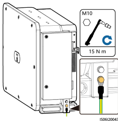
Abbildung 5-11 Kabelanschluss
