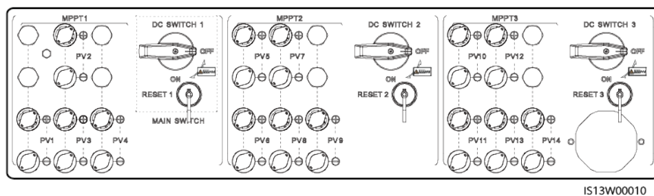
Abbildung 5-15 DC-Klemmen
