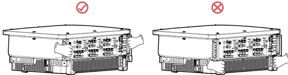
Abbildung 4-12 Hebeposition
