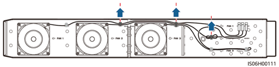
Abbildung 8-7 Entfernen der Kabelbinder für LÜFTER 2
