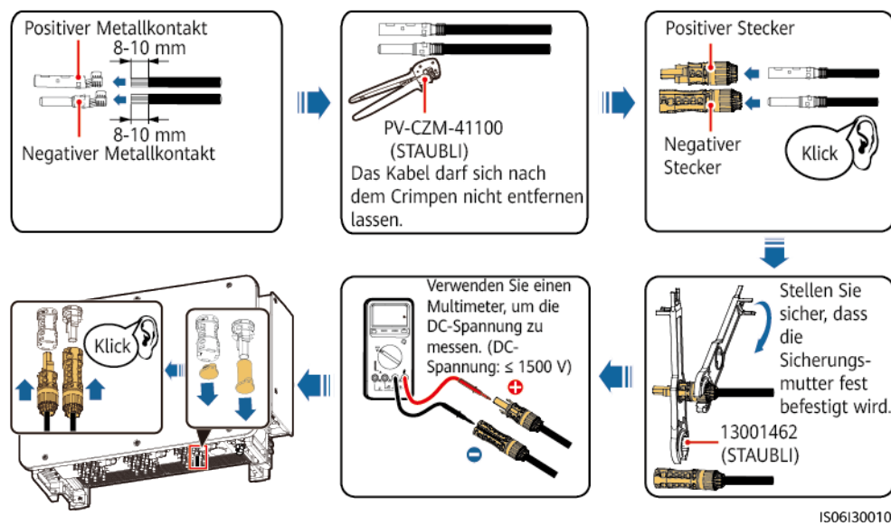
Abbildung 5-16 Kabelanschluss
