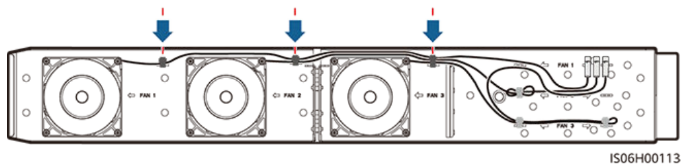
Abbildung 8-11 Zusammenbinden der Kabel für LÜFTER 1
