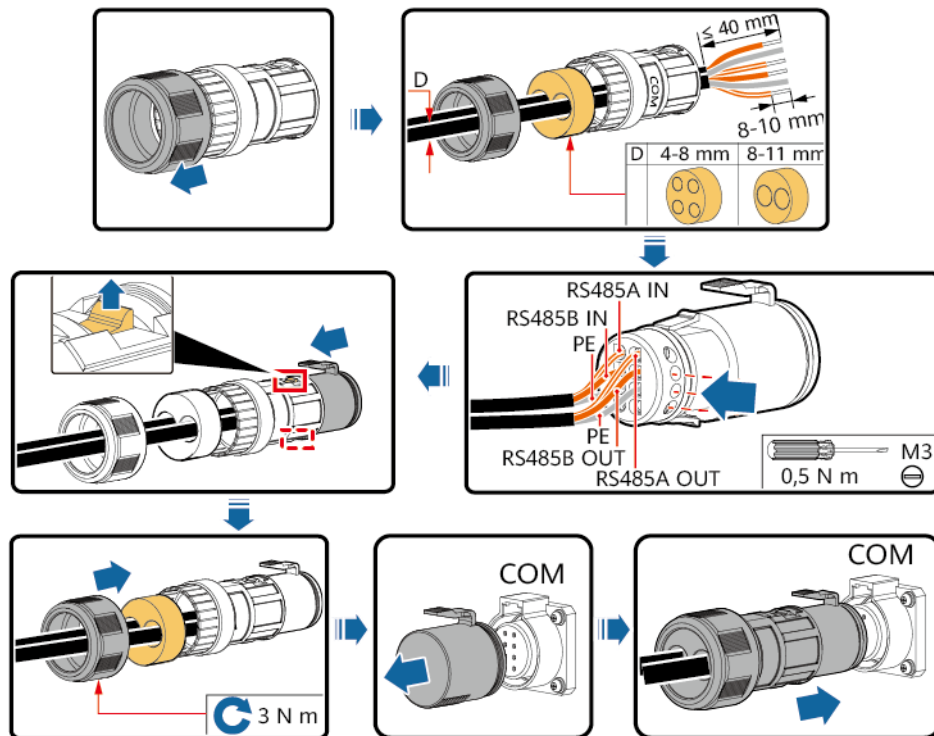
Abbildung 5-20 Kabelverbindung (vierlöchriger Gummistöpsel 4-8 mm)
