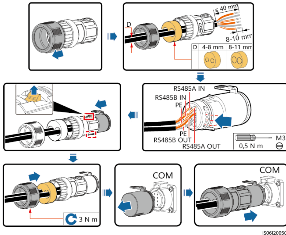
Abbildung 5-21 Kabelverbindung (zweilöchriger Gummistöpsel 4-8 mm)
