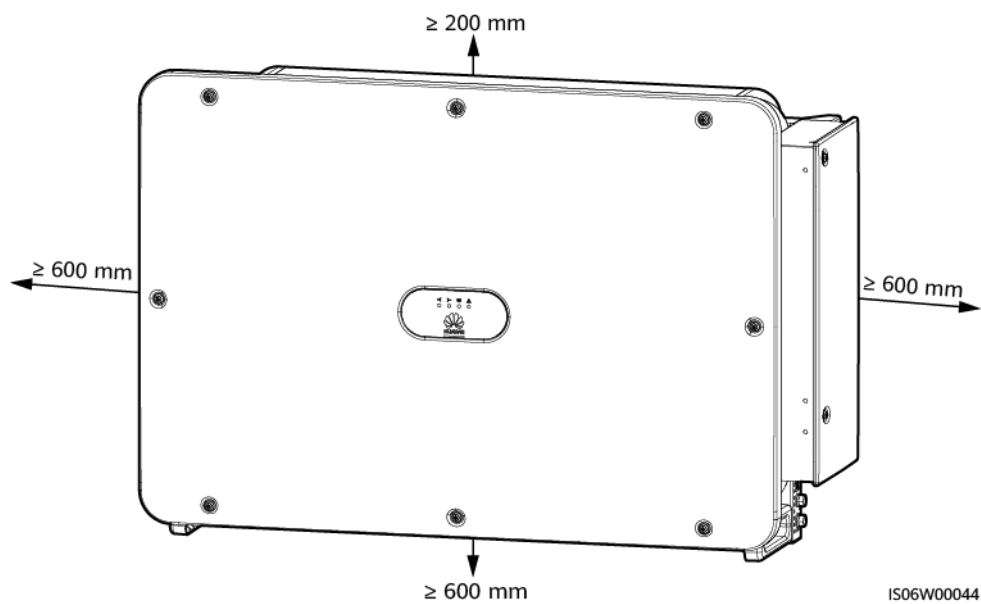
Abbildung 4-2 Montageabstände
